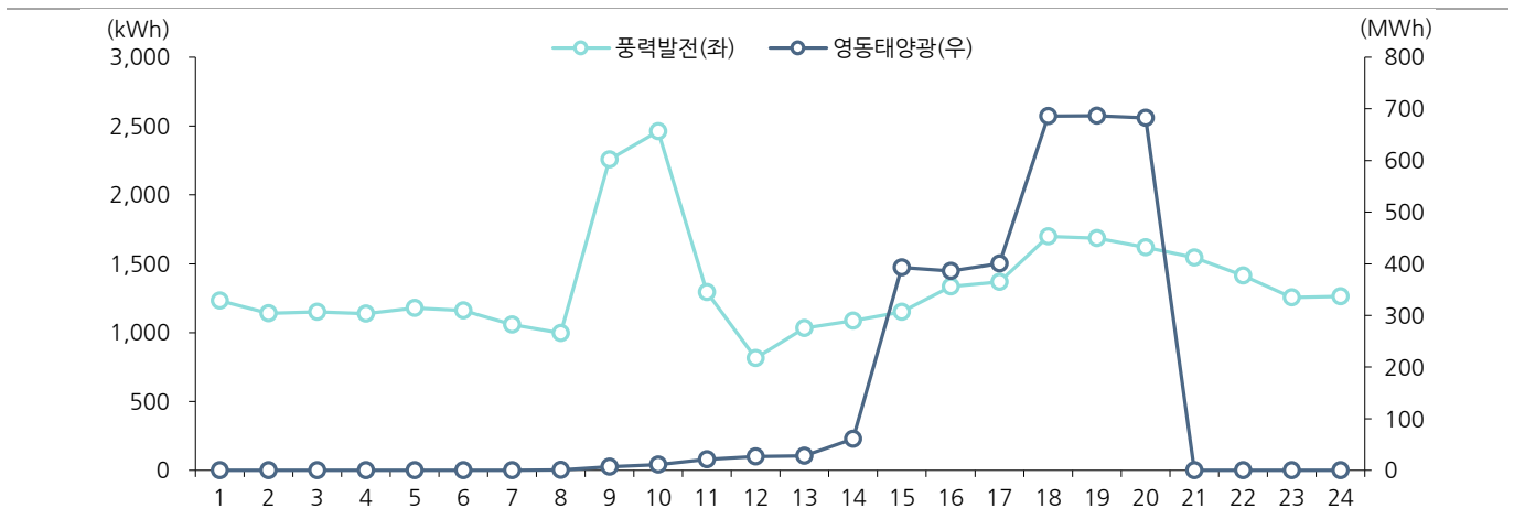
그림41. 풍력발전 및 태양광발전 시간대별 발전량
