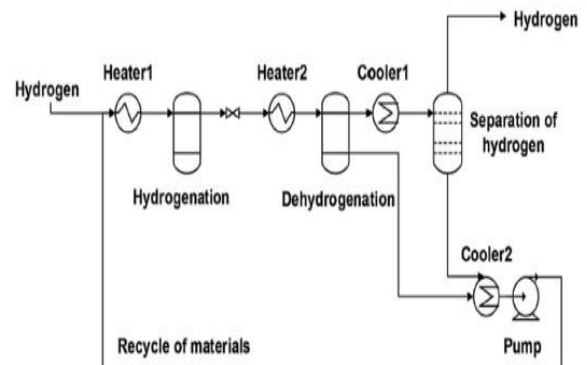
그림55. LOHC를 이용한 수소 저장/배출 공정의 예
