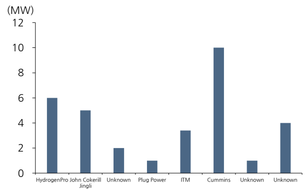
그림83. 2022 아시아태평양 공급자별 수전해설비 출하량(단위 : MW, ex-China)
