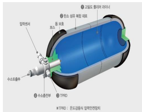
그림61. 수소공급방식 : 수소탱크
