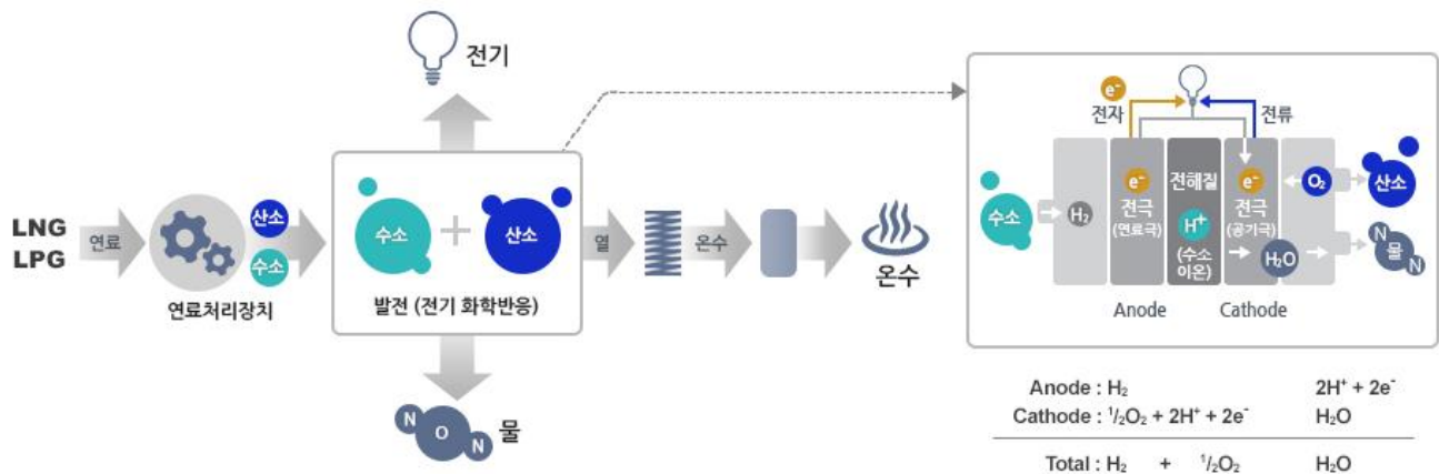
그림59. 수소연료전지 구조
