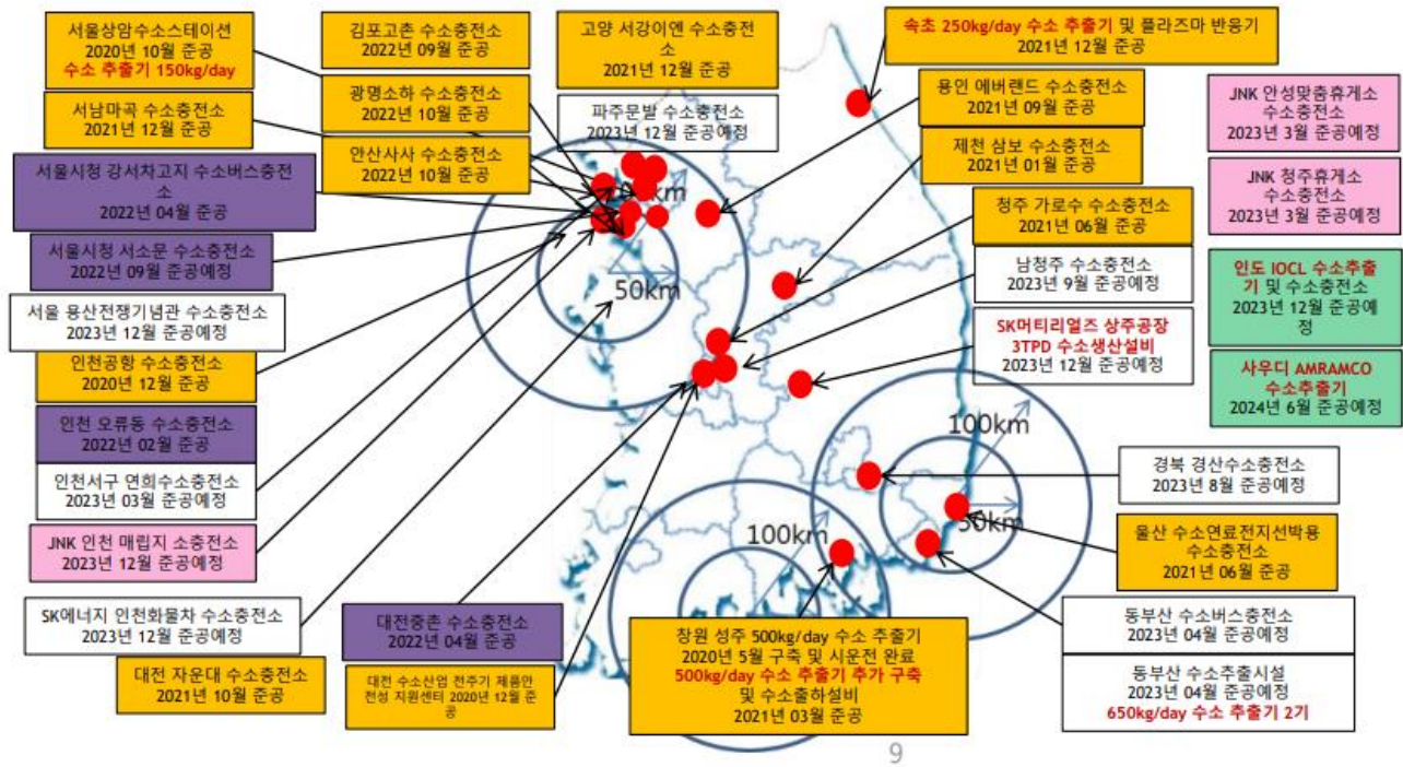
그림 8. 제이엔케이히터 수소충전소 구축현황
