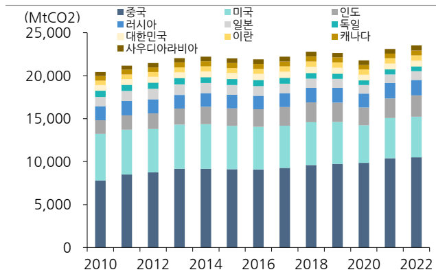
그림 2. 국가별 연료 연소로부터의 이산화탄소 배출량 추이
