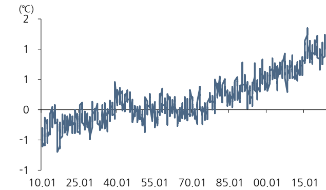
그림 1. 글로벌(Land&amp;Ocean) 1901~2000 100년 평균 기온 대비 편차
